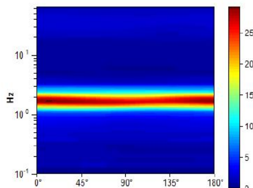
DIREZIONALITA' H/V
